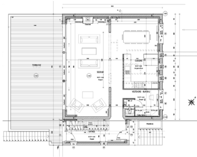
Rez-de-chaussée (extension)
