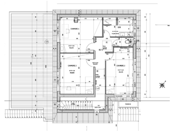
R+1 (surélévation)
